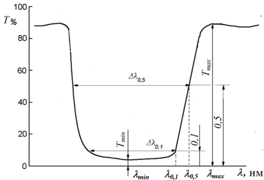
Рис. 1. Основні характеристики відрізаючих оптичних фільтрів
