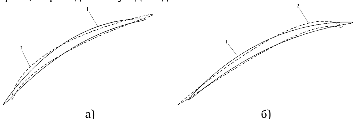
Рис. 2. Зміна положень профілю лопатки при додатному та від'ємному значенні параметра \alpha у виразі (3): а) 1 – початкова форма профілю при \alpha = 0 ; 2 – форма профілю при \alpha = 0,7 ; б) 1 – початкова форма профілю при \alpha = 0 ; 2 – форма профілю при \alpha = -0,7
