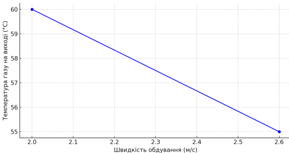
Рис. 1. Залежність температури коксового газу на виході від швидкості обдування
