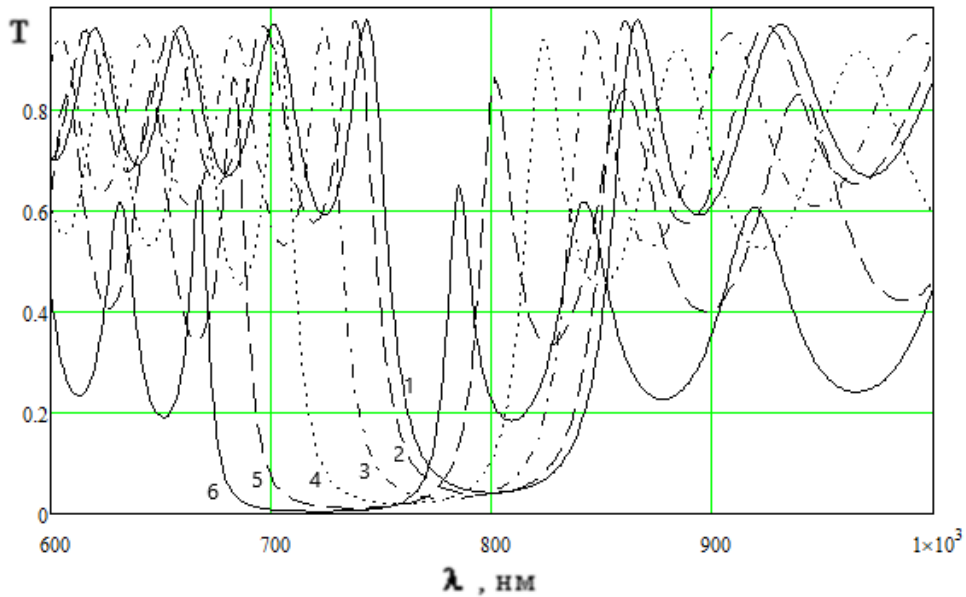
Рис. 2. Трансформація спектрів пропускання 25-шарового відрізаючого оптичного фільтра з робочою довжиною хвилі \lambda_0 = 800 нм для s -поляризації при зміні кута падіння: 1- \theta_0 = 0^\circ ; 2 - \theta_0 = 15^\circ ; 3 - \theta_0 = 30^\circ ; 4 - \theta_0 = 45^\circ ; 5 - \theta_0 = 60^\circ ; 6 - \theta_0 = 75^\circ
