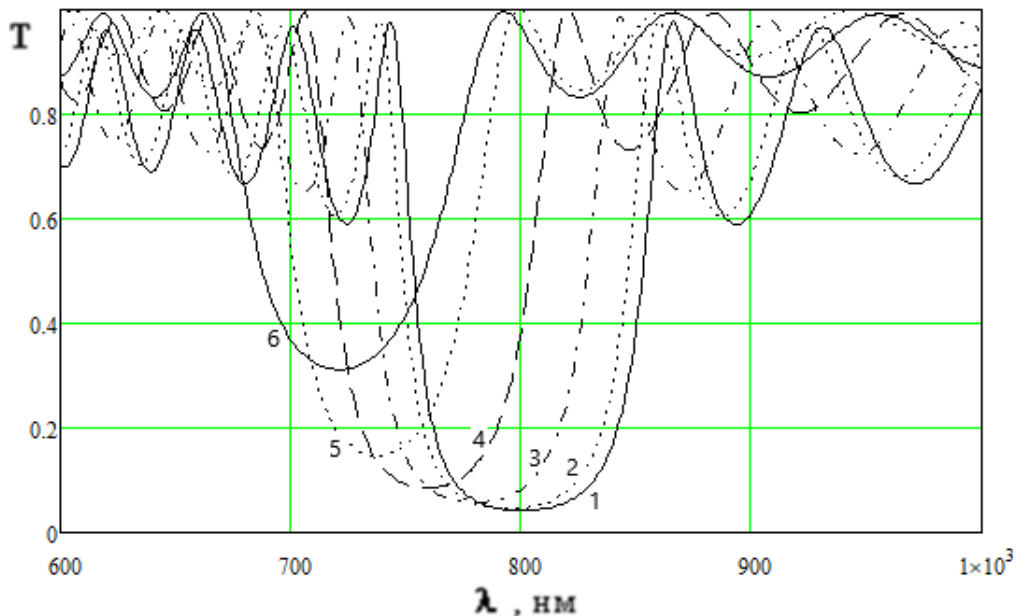
Рис. 3. Трансформація спектрів пропускання 25-шарового відрізаючого оптичного фільтра з робочою довжиною хвилі \lambda_0 = 800 нм для p -поляризації при зміні кута падіння: 1- \theta_0 = 0^\circ ; 2 - \theta_0 = 15^\circ ; 3 - \theta_0 = 30^\circ ; 4 - \theta_0 = 45^\circ ; 5 - \theta_0 = 60^\circ ; 6 - \theta_0 = 75^\circ
