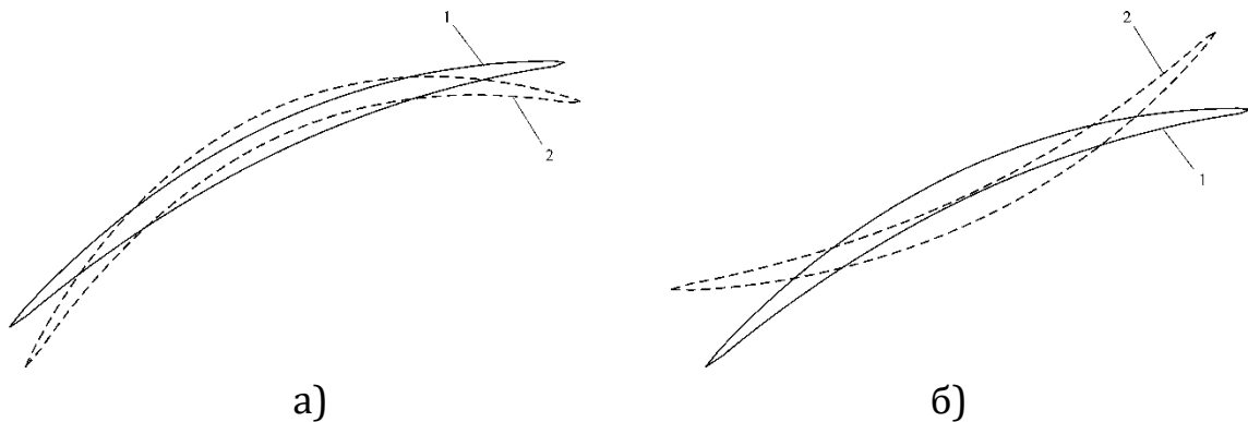
Рис. 1. Зміна положень профілю лопатки при додатному та від'ємному значенні параметра \xi у виразі (2):
